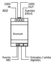
Conexión Módem monofásico
