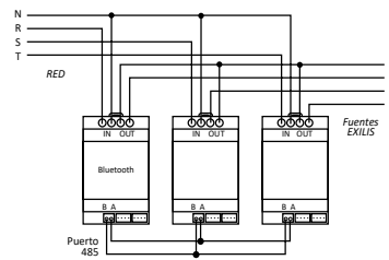
Conexión Módem trifásico
